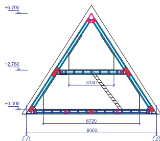
Разрез
