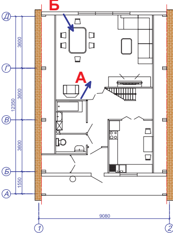
План 2 этажа
